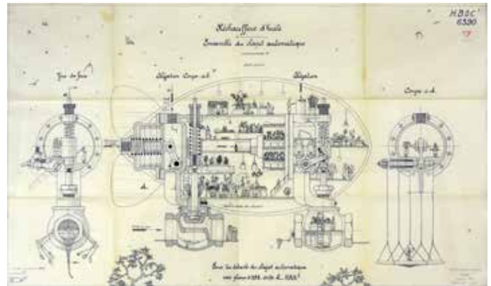
Plan 6 : Réchauffeur d'huile.
